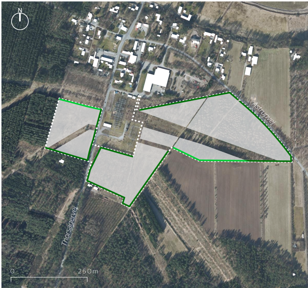
Kort 7.10: Med lys grøn linje vises princippet for etablering af beplantningsbælter omkring solcelleområdet. Med mørk grøn linje vises princippet for supplering og bevaring af eksisterende beplantningsbælter. Plan- og projektområdet er vist med hvid linje omkring de lyse grå flader der udgør byggefeltet til solcelle paneler.
