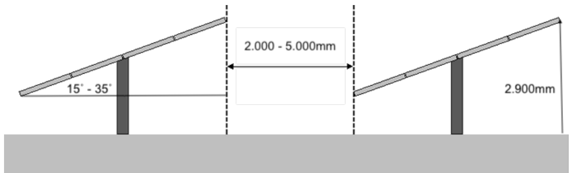
Figur 9: typisk arrangement af solcellepaneler
