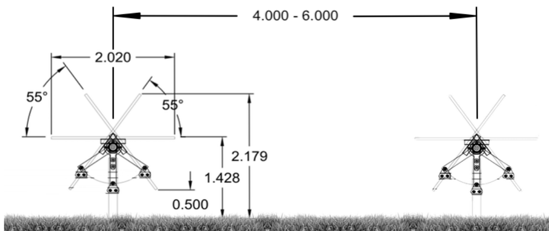
Figur 10: Dynamisk arrangement af solcellepaneler
